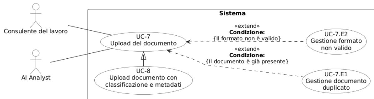
Figura 52: Diagramma del caso d'uso UC-7: Upload del documento
